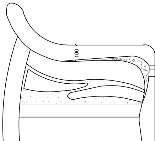
沙发侧立面图 SCALE 1:10
